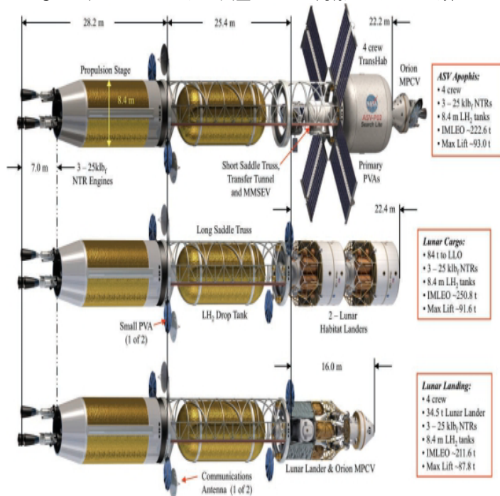
図 地球に近い小天体を探査する宇宙船の概念 (48th Joint Propulsion Conference & Exhibit, Atlanta, GA, July 30 - August 1, 2012) (SEJ注：火星へのほぼ同様のシステムで探査)
