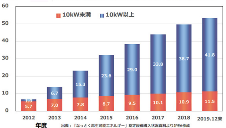
(GW) 日本の太陽光発電の導入状況：累積導入量
